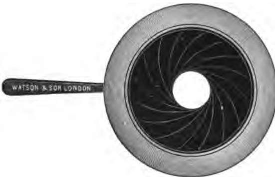
FIG. 46.—Iris diaphragm.
